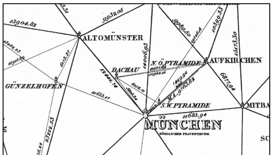
Hauptdreiecksnetzpunkte in Bayern (Ausschnitt), Quelle: Bayerische Vermessungsverwaltung.
